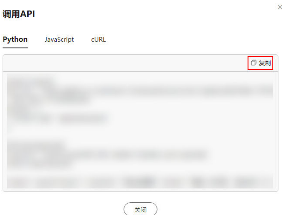
图 1-8 调用接口
